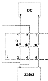
Zapojení pro DC obvody
